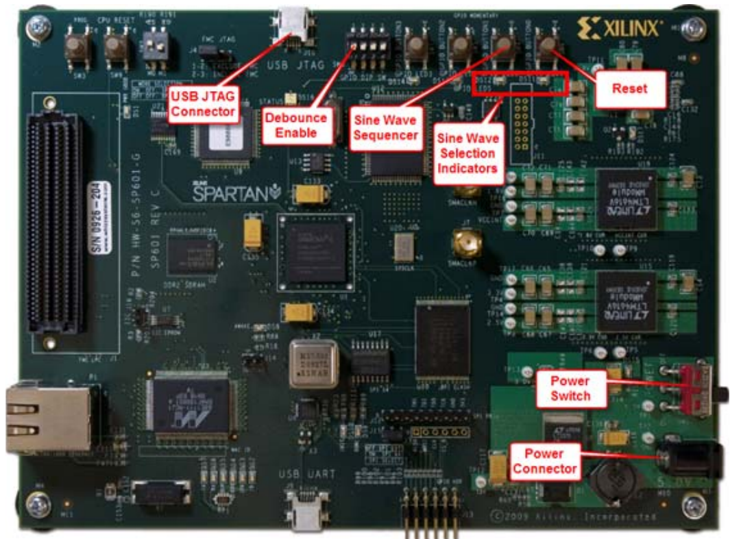
図 1 : SP601 ボード
