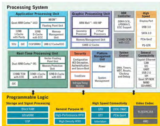
图 2：MPSoC 原理图
