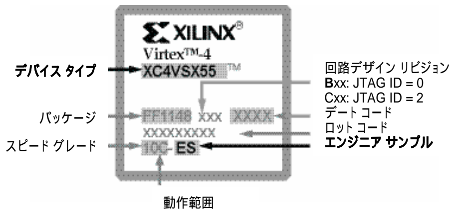
図 1: XC4VSX55CES パッケージ マーク例
