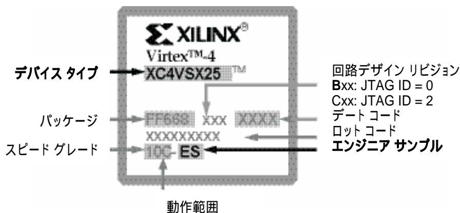
図 1: XC4VSX25CES パッケージ マーク例
