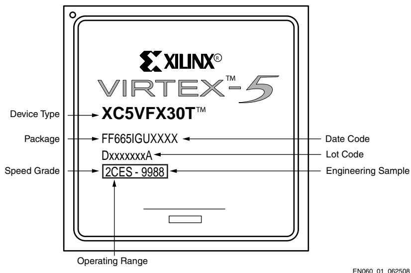
図 1: XC5VFX30T CES9988 のパッケージ マーク例
